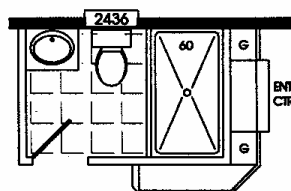
OPTIONAL 60" SHOWER
